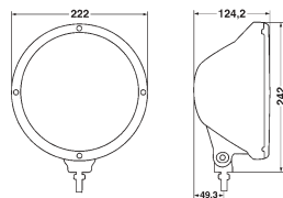
Montaggio a sbalzo: ritto. Angolo di inclinazione da -45° a +90°
