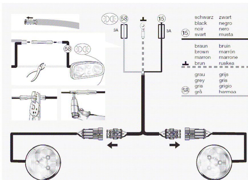
Fig: Elektrisk tilslutning
