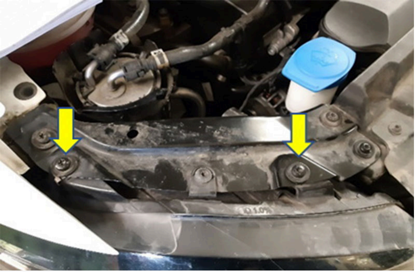
Sabitleme vidalar#
