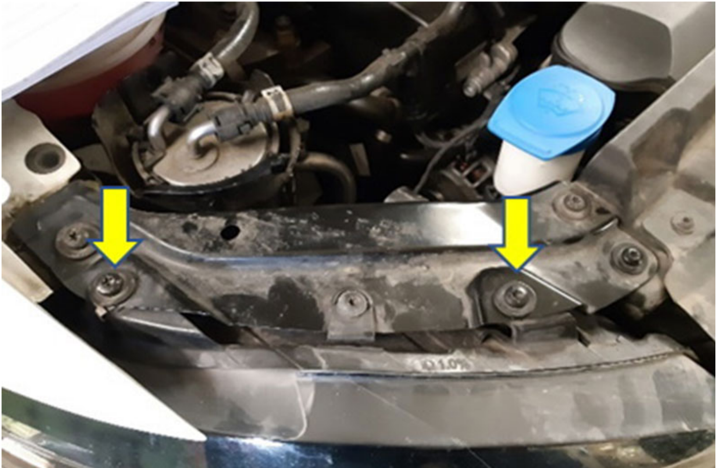
Bevestigingsbouten
