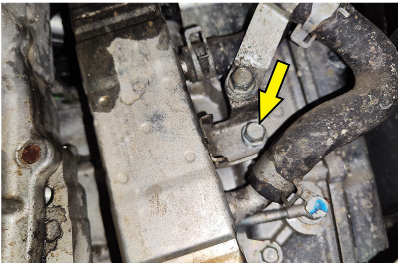
Subaru Forester EGR-koeler schroef onder
