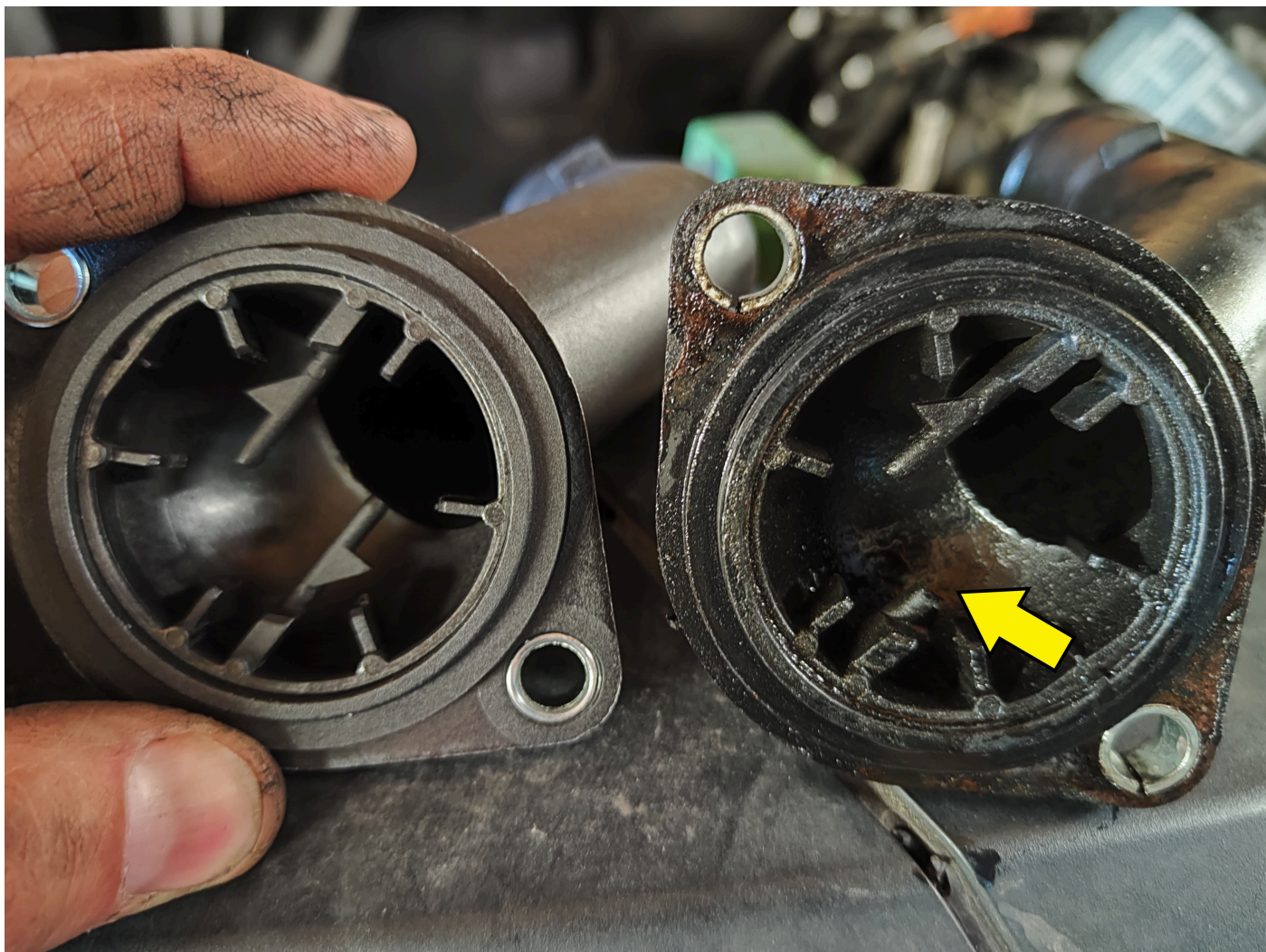
Guida in plastica della flangia del liquido di raffreddamento T5
