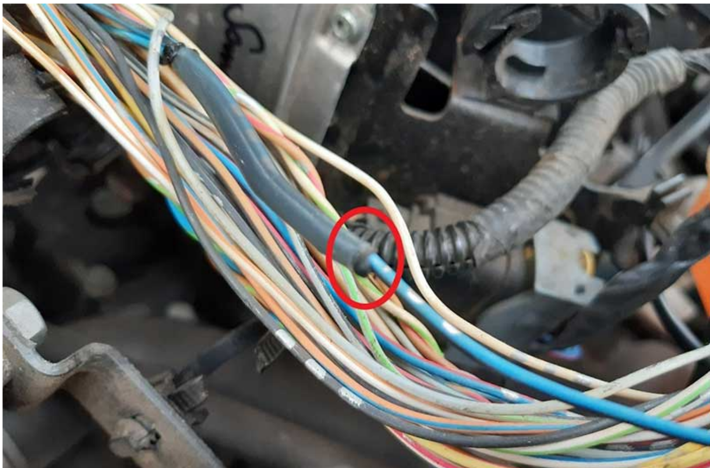
Figure 2 : Les vibrations peuvent casser le câble à certains endroits
