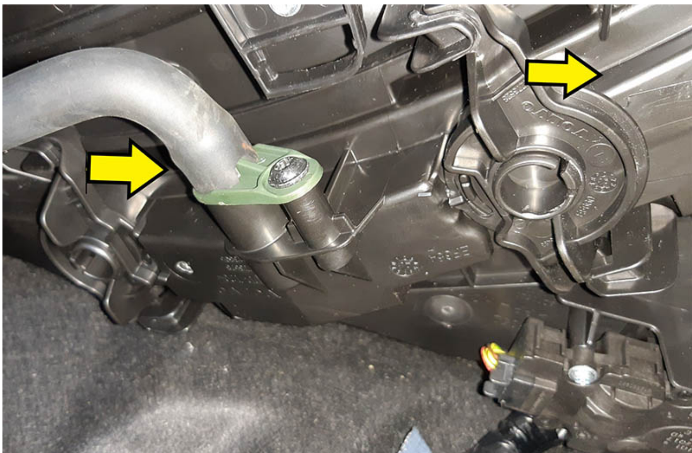
Revestimiento espacio reposapiés
