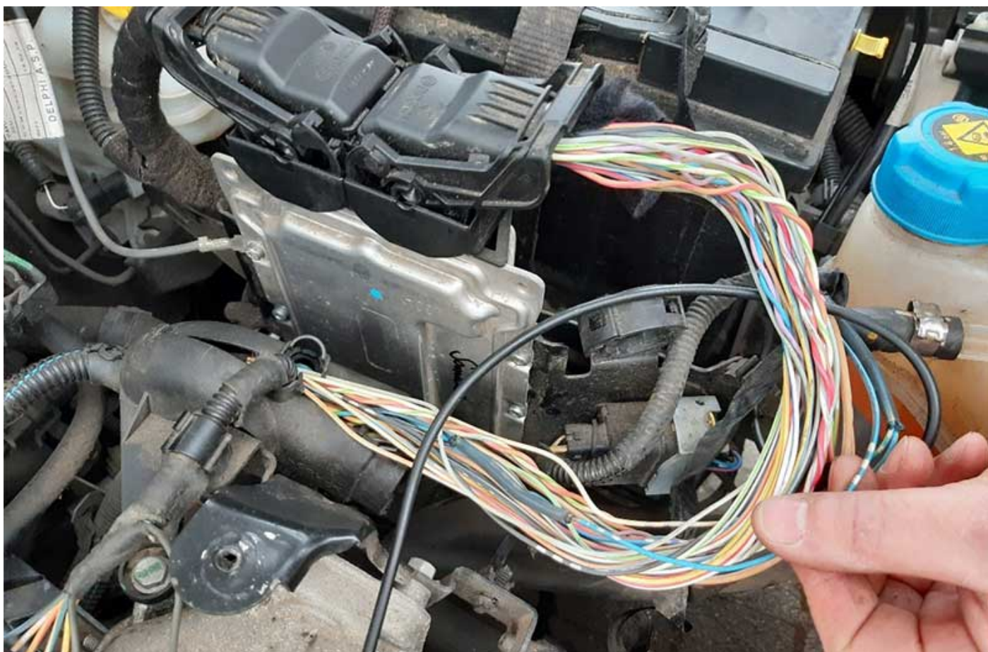
Fig. 1: Kontroller ledningsnettet, der fører fra motorstyringsenheden til tændspolen eller indsprøjtningsdyserne
