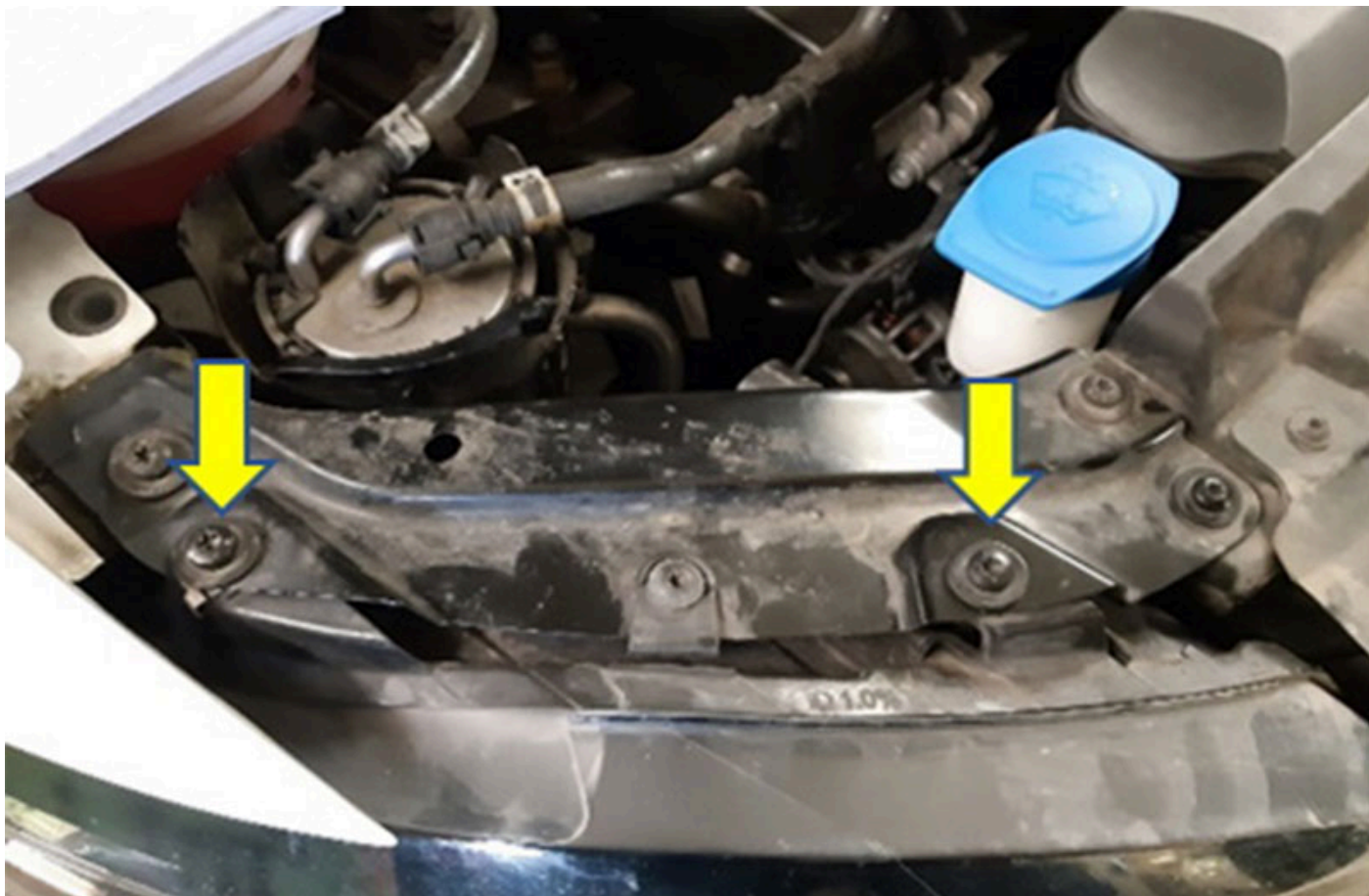
Vis de fixation
