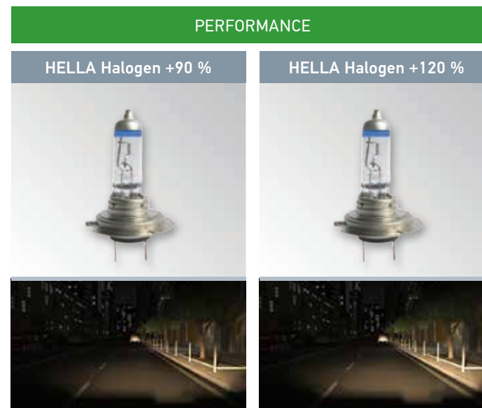
Ausleuchtung +90 %
