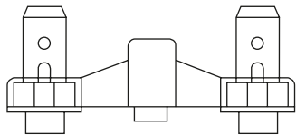
Desenho ligação A Conector plano com 6,3 mm, zincado
