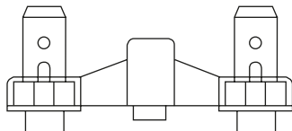
Tekening aansluiting A 6,3 mm vlakke stekker, verzinkt
