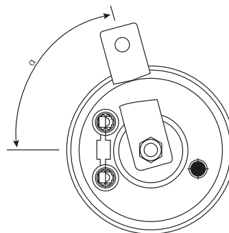
Tegning holdeposition (vist som eksempel)
