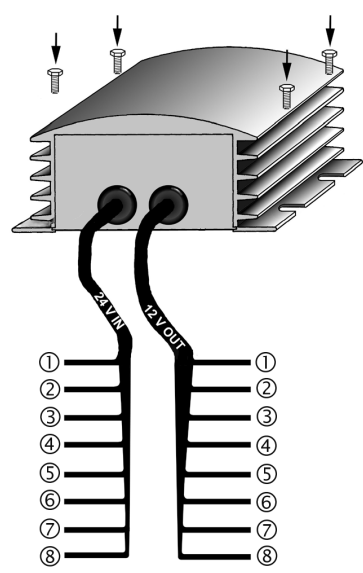
Elektrischer Anschluss 5DS 008 125-011
