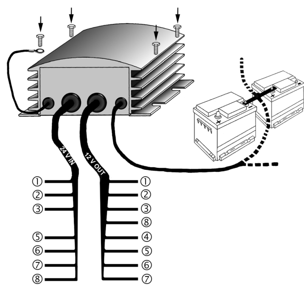
Elektrischer Anschluss 5DS 008 125-001
