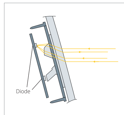
Frontlichtsensor
