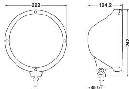
Anbau: Stehend. Neigungswinkel -45^\circ bis +90^\circ
