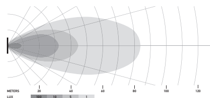
Set LED Cube 3,2", proiettore
