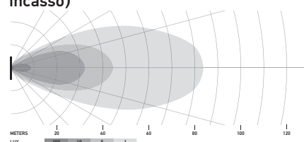
Set LED Cube 3,2", proiettore (a incasso)
