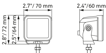
LED Cube 3,2" (version pour montage en saillie)
