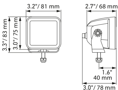
LED Cube 3,2" (version pour montage en saillie)
