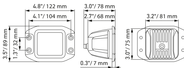
LED Cube 3,2" (version pour montage encastré)
