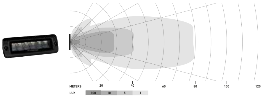
Black Magic Mini Lightbar 6,2", montaje empotrado, luz difusa
