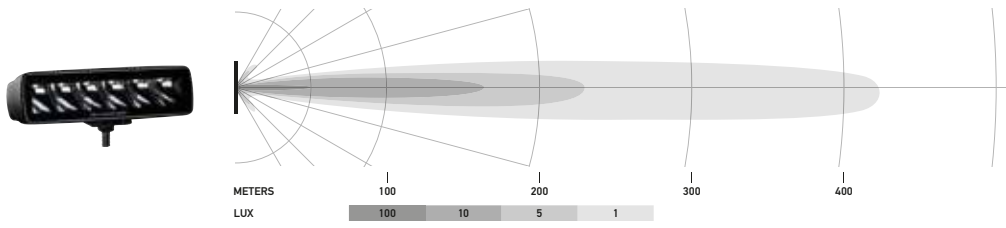
Black Magic Mini Lightbar 6,2", haz de luz puntual
