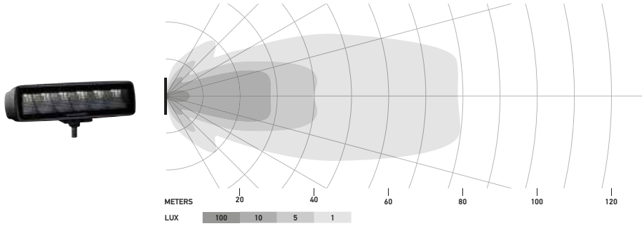
Black Magic Mini Lightbar 6,2", luz difusa
