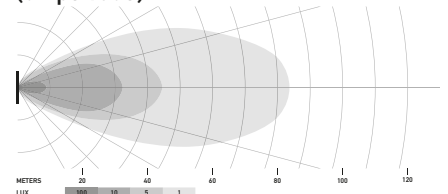
LED Cube SET 3,2", luz difusa (empotrado)
