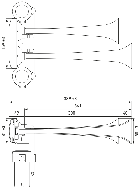
CA44 verchromde dubbele claxon
