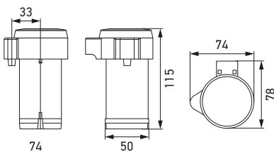
Vervangend onderdeel | CM40 compressor
