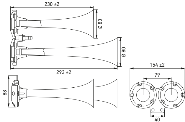
CA42 verchromde dubbele claxon
