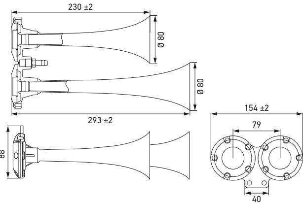
CA42 Krom dobbelt lufthorn
