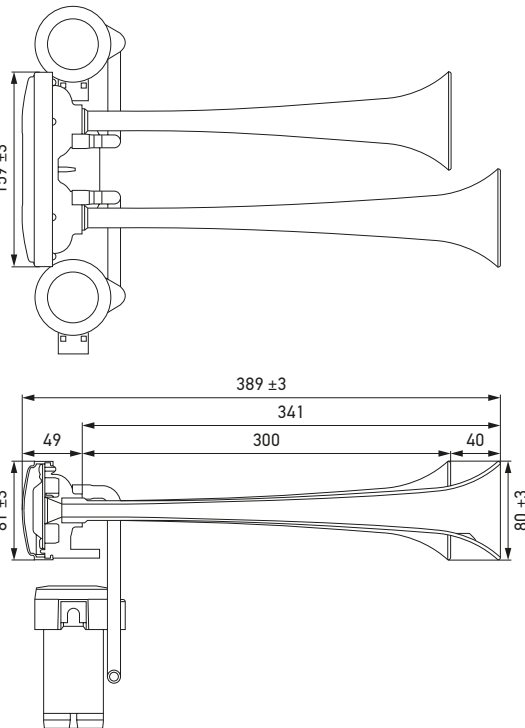
CA44 Krom dobbelt lufthorn
