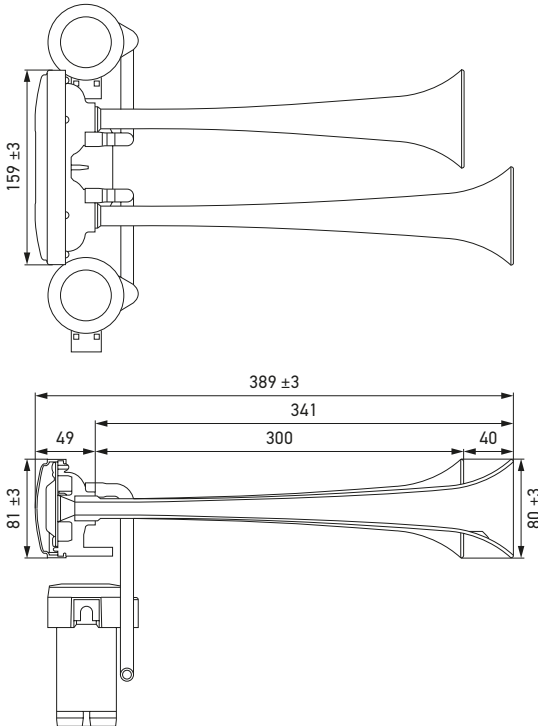
CA44 Doppel-Druckluftfanfare, Chrom
