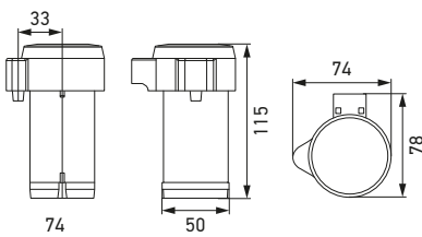
Ersatzteil | CM40 Kompressor
