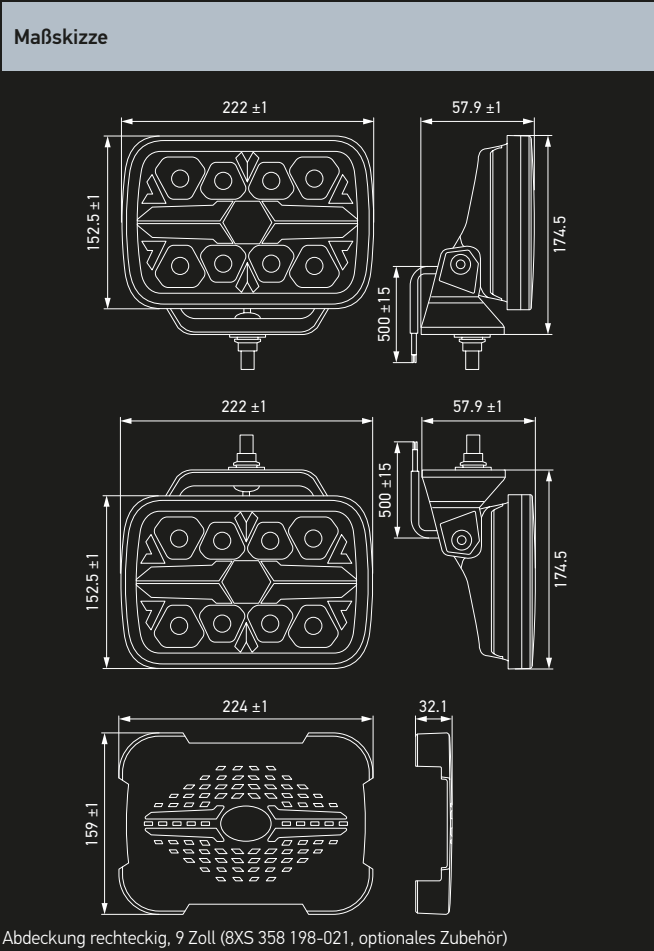
Abdeckung rechteckig, 9 Zoll (8XS 358 198-021, optionales Zubehör)
