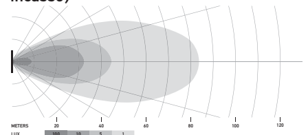
SET LED Cube 3.2", proiettore (a incasso)
