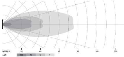
SET LED Cube 2.7", proiettore
