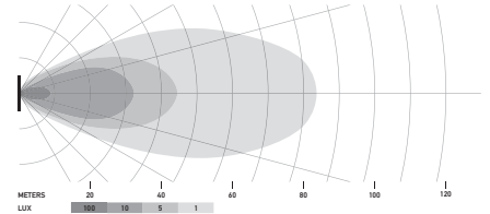
SET LED Cube 3.2", proiettore
