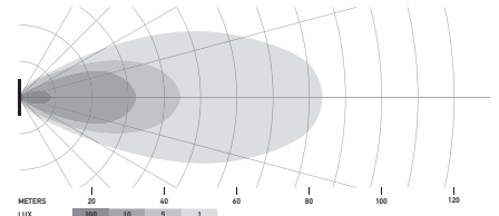
LED Cube SET 3,2", Flutlicht (Einbau)
