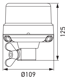
Rohrstutzen-Befestigung
