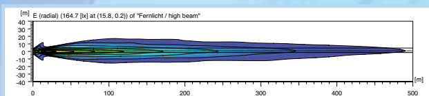
Rallye 3003 (Rif. 37,5) con riflettore High Boost
