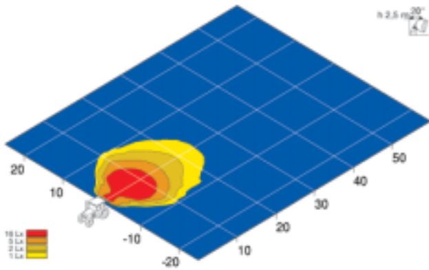
Objektbelysning 20°
