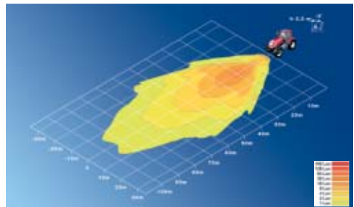
Terrænbelysning 5°
