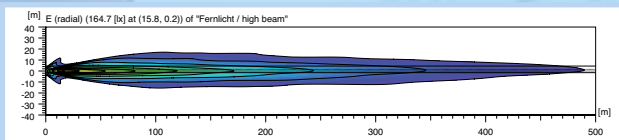
Rallye 3003 (Réf. 37,5) avec réflecteur de précision
