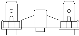
A bağlantısı çizimi 6,3 mm düz fiş, bakır
