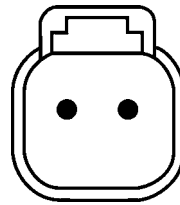
E bağlantısı çizimi Sıçrama suyu korumalı DEUTSCH fiş DT 06-25
