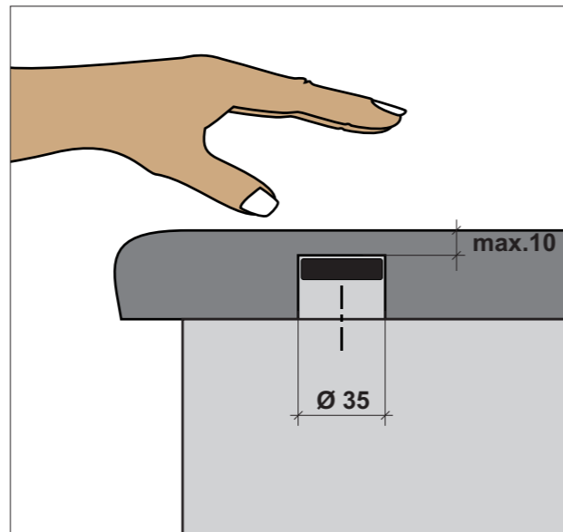
Prinzip des berührungslosen Schaltens
