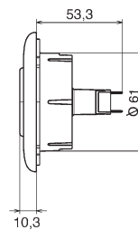
Einbau, verstellbar
