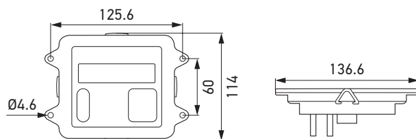
Steuergerät
